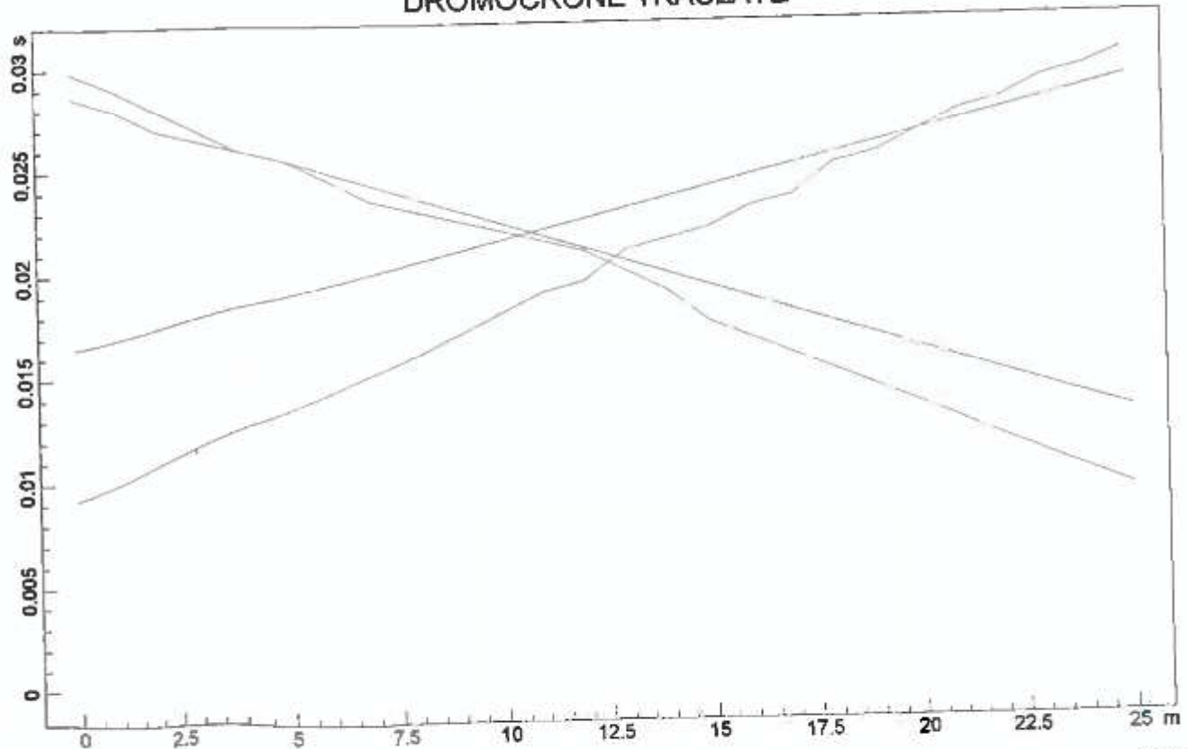
DROMOCRONE TRASLATE
