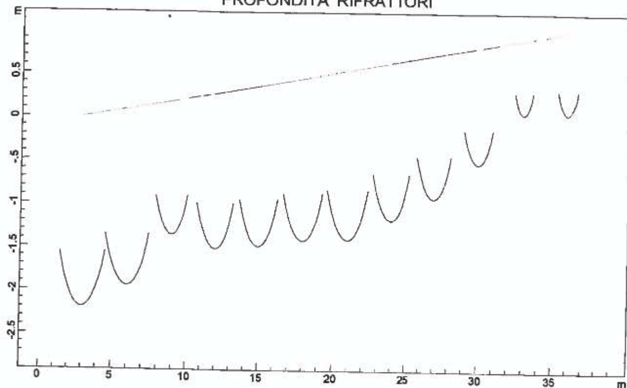
PROFONDITA' RIFRATTORI
