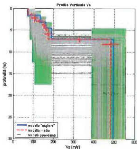
curve di dispersione: spettro.cdp VS30 (modello "migliore"): 292 m/s VS30 (modello medio): 280 m/s
