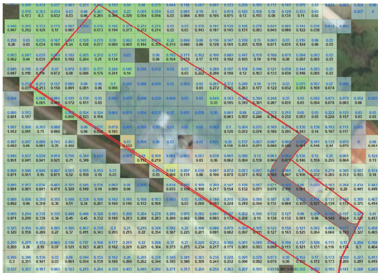
Figura 8-6: Perimetro del PUC R5 e indicazione delle celle di calcolo con i valori di battenti (espresso in metri) nelle configurazioni di progetto (valori di colore nero) e di stato attuale (valori di colore blu).
