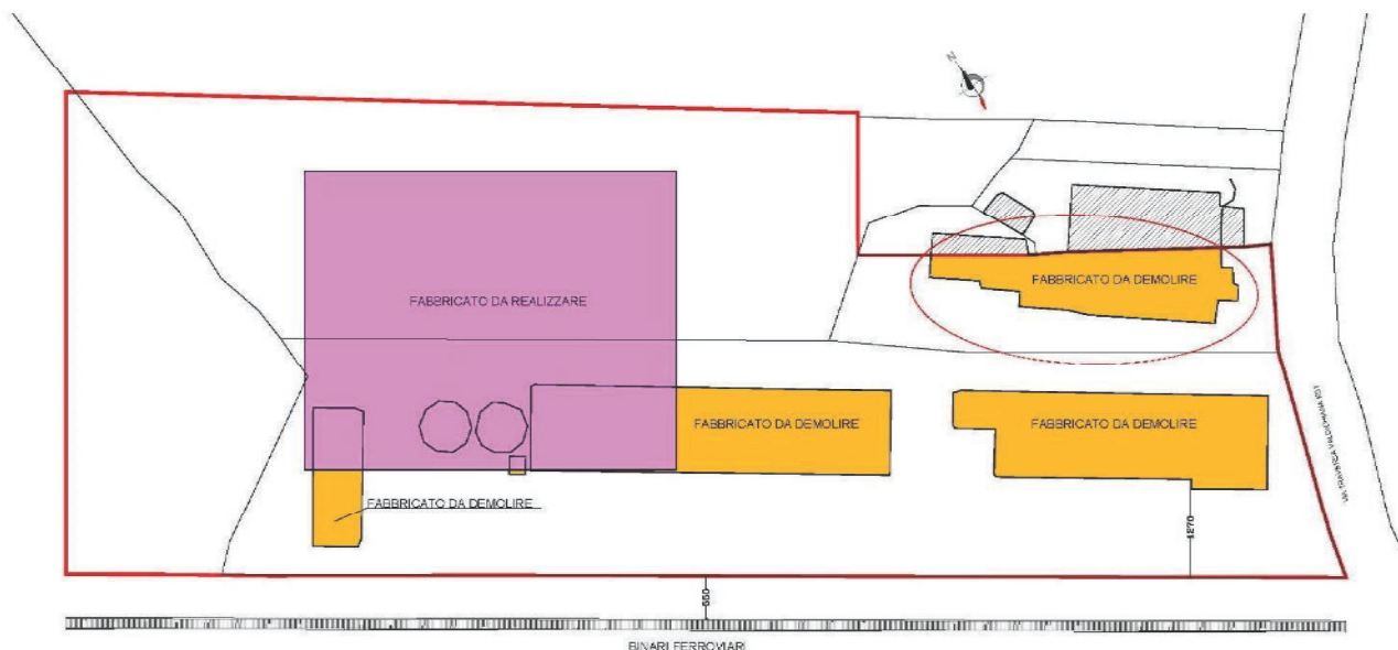
Figura 8-2: Planimetria con rappresentazione del perimetro della previsione PUC R5, dei fabbricati esistenti da demolire e dell'area in cui è prevista la realizzazione di un nuovo fabbricato
