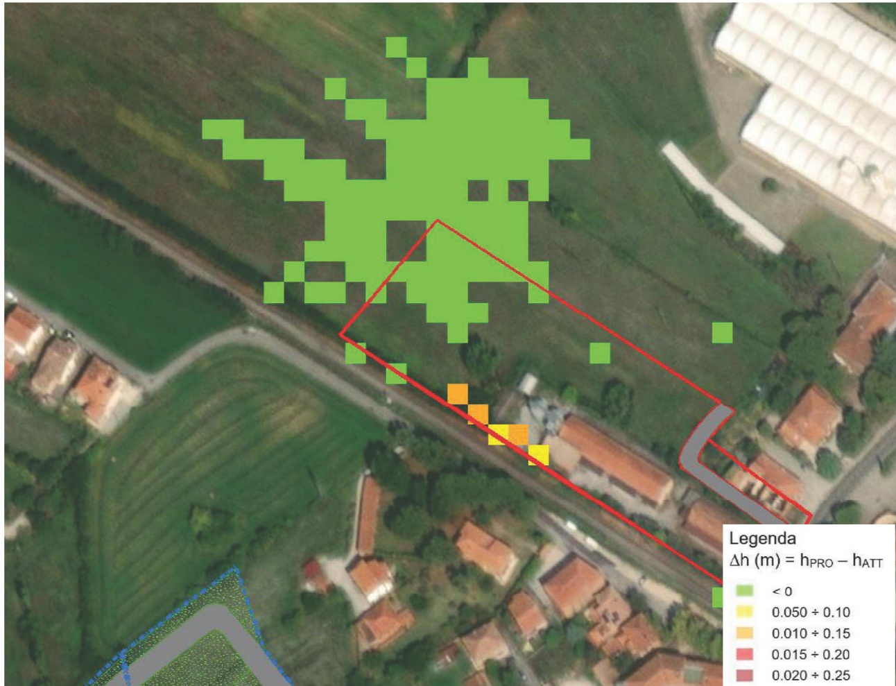
Figura 8-5: Perimetro del PUC R5 e indicazione delle celle di calcolo in cui si è calcolato una variazione di battente idraulico nello scenario di progetto rispetto allo scenario di stato attuale.
