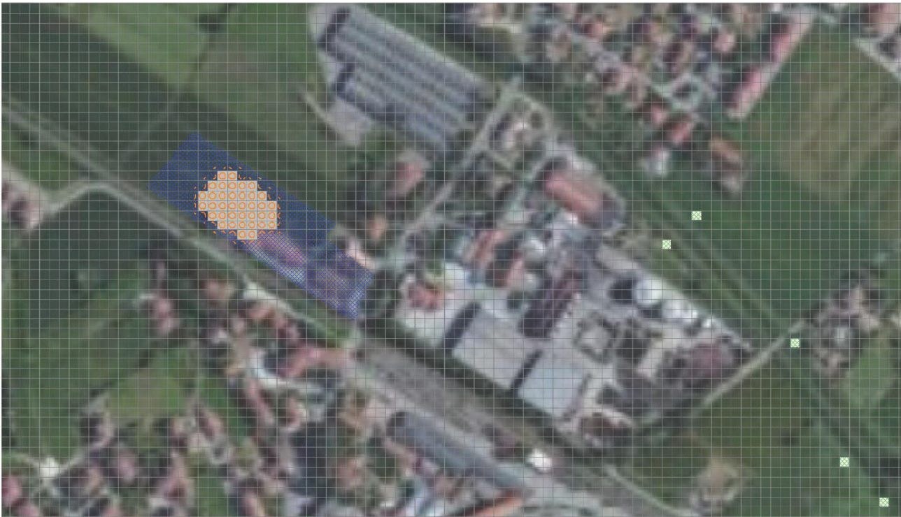
Figura 8-4: Perimetro del PUC R5 con rappresentazione delle celle "ostruite" nello scenario di progetto per simulare la realizzazione della sopraelevazione su rilevato.
